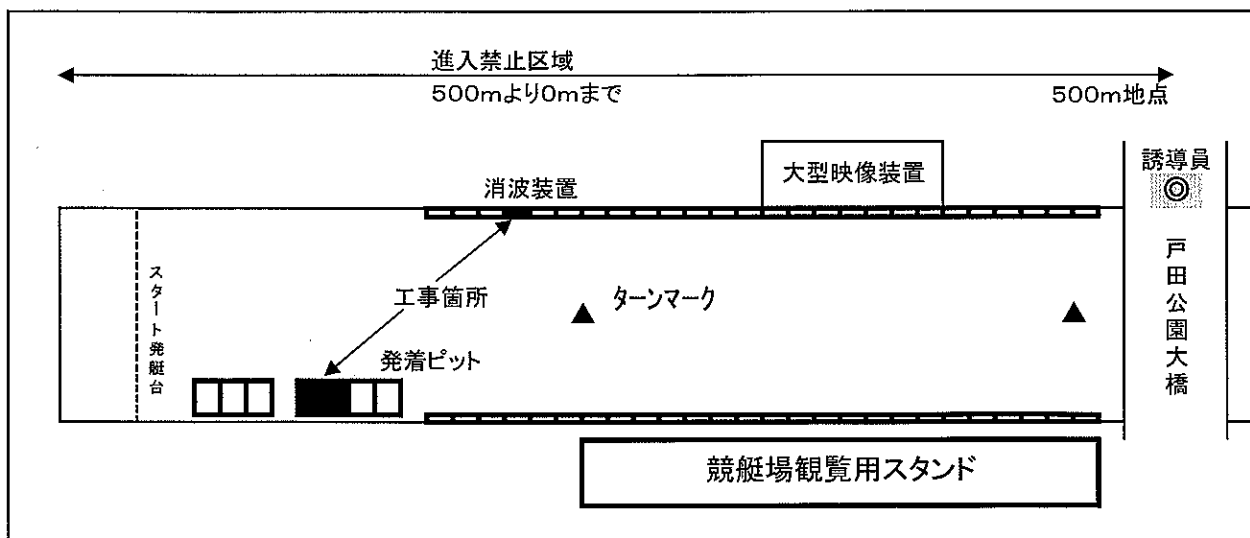
工事図
